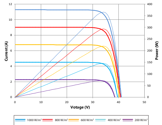
电流-电压 & 功率-电压曲线图 (370S)
